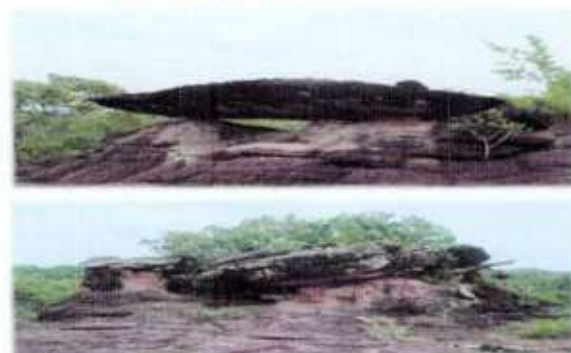
กลุ่มหินเทิบ กลุ่มที่ ๒ (ห่างจุดชมวิวประมาณ ๕๐๐ เมตร)
